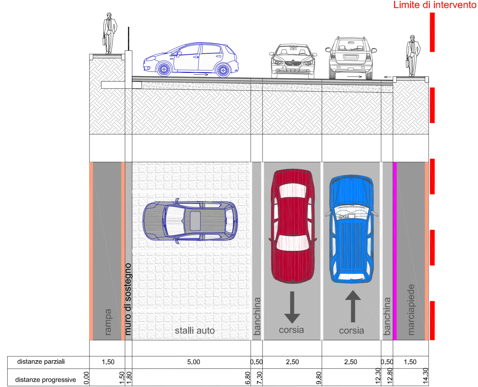
Sezione tipo D-D'
