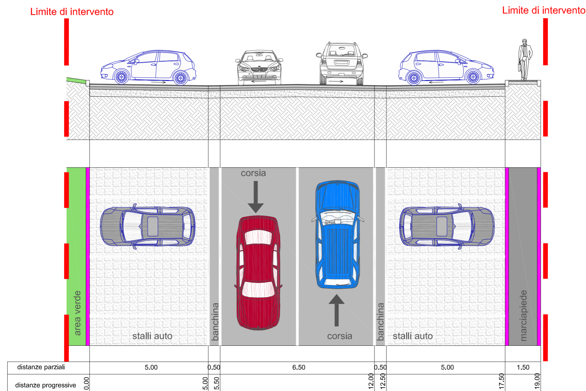
Sezione tipo B-B'
