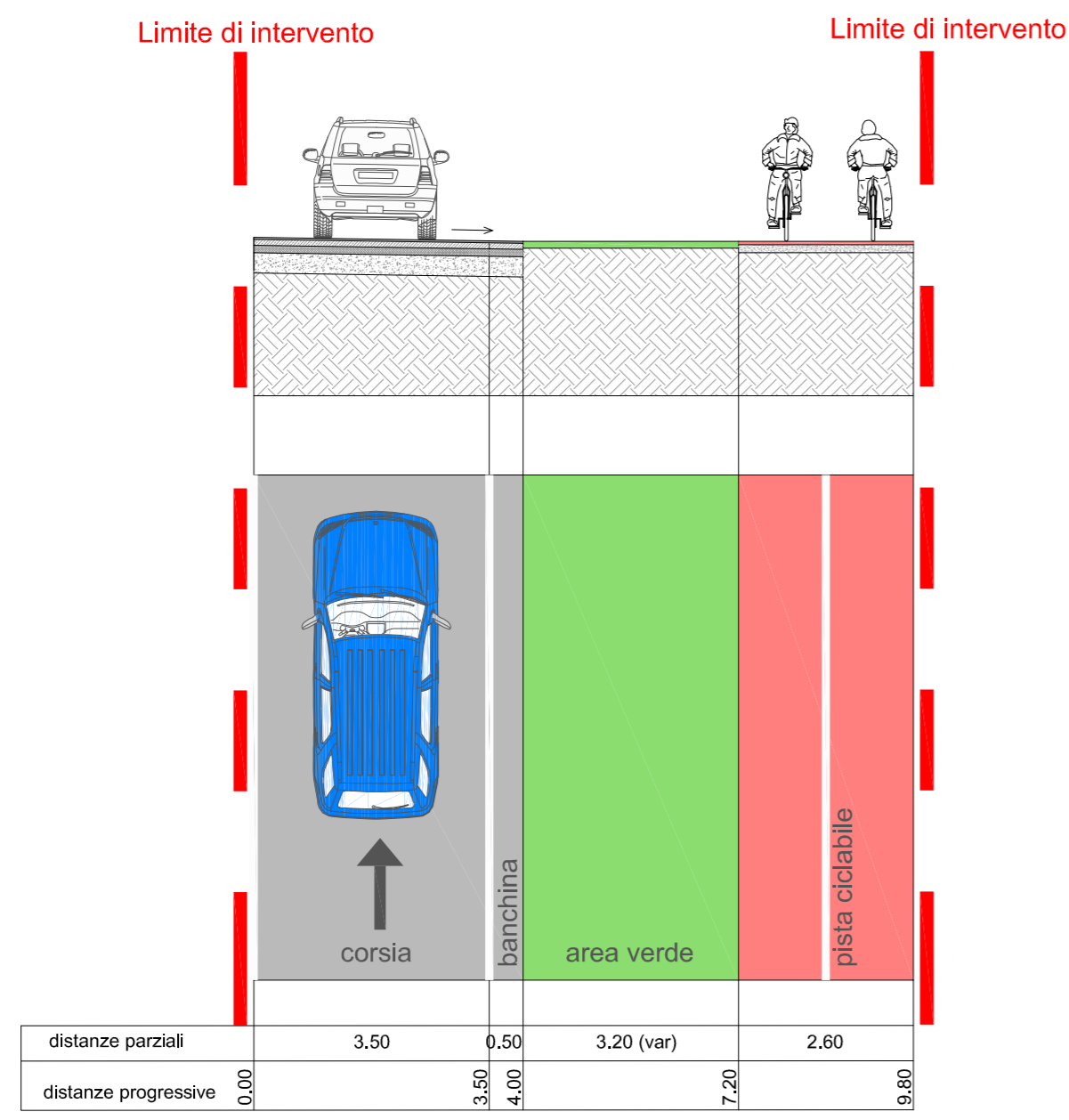
Sezione tipo B-B'
