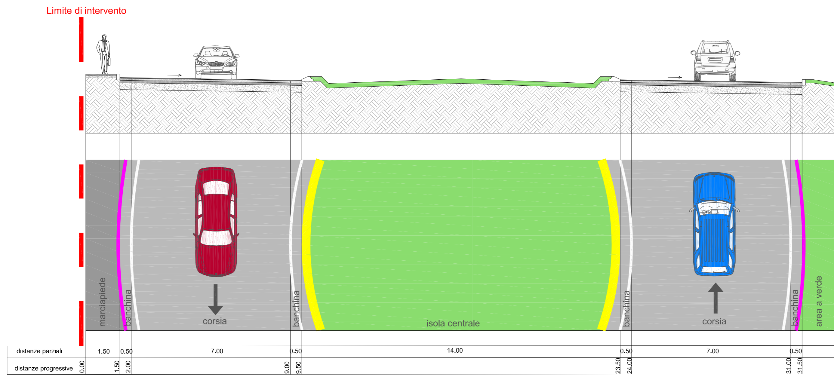
Sezione tipo A-A'
